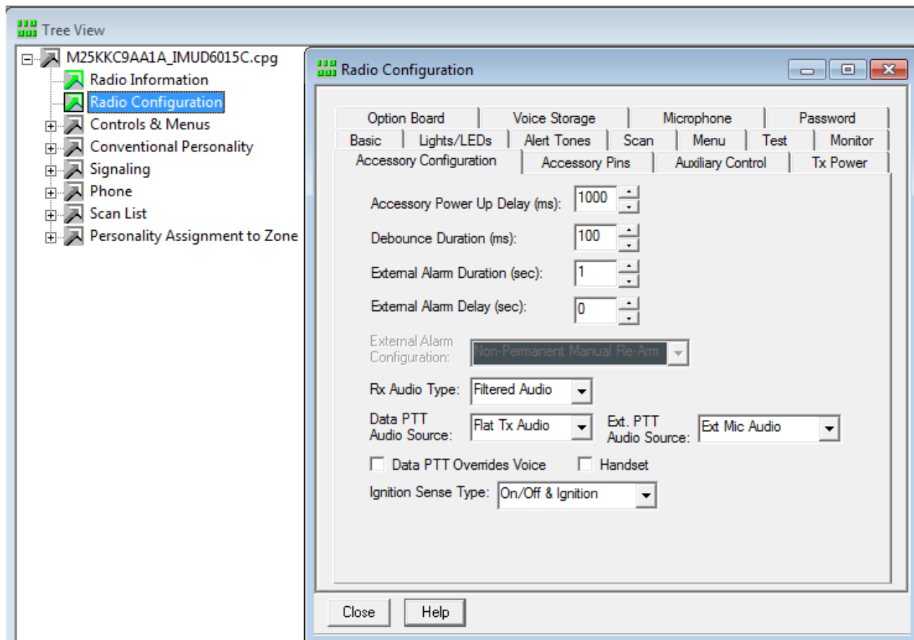
Рис.5.2.2.3.1 Окно «Radio Configuration», панель «Accessory Configuration».
