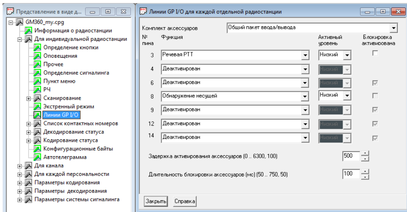
Рис.5.2.2.4.3 Окно «Линии GP/IO», установка функций контактов аксессуарного разъёма.
