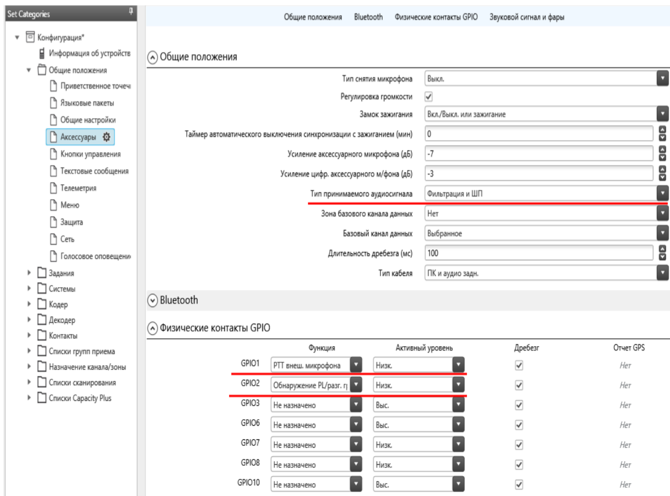
Рис. 5.2.2.6.2 Окно «Аксессуары» программы «MOTOTRBO CPS» версии 2.0 (2020г).
