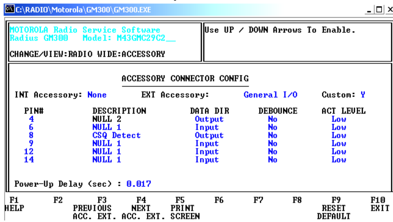
Рис.5.2.2.1.2 Окно «ACCESSORY CONNECTOR CONFIG».
