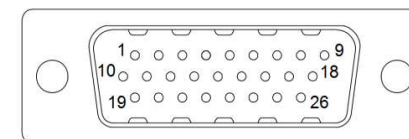
Разъем DHS-26M (вид спереди)
