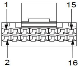
Разъем HLN9457 (вид спереди)
