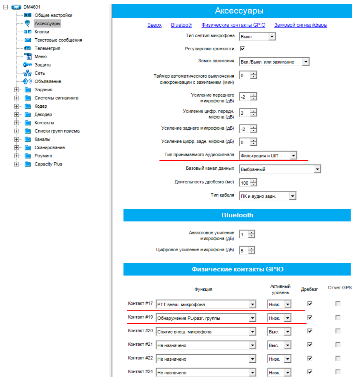
Рис. 5.2.2.6.1 Окно «Аксессуары» программы «MOTOTRBO CPS» версии 15.5 (2017г).
