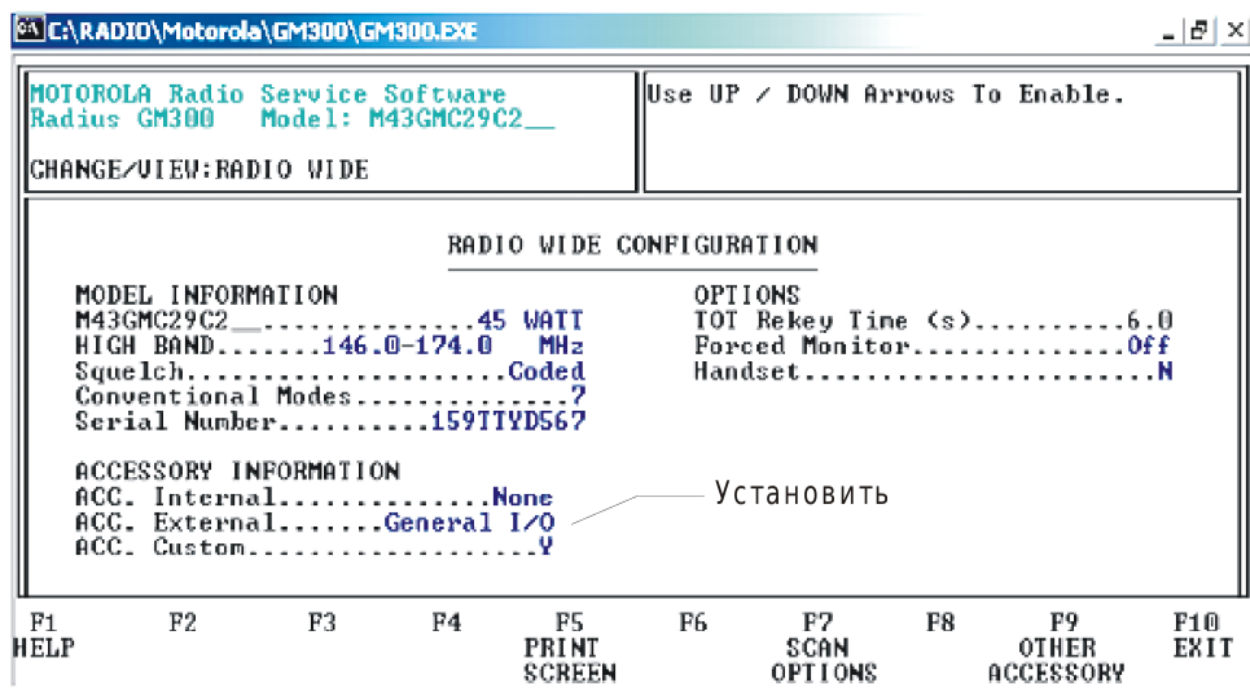
Рис.5.2.2.1.1 Окно «RADIO WIDE Configuration: Scan, Accessory Connector».
