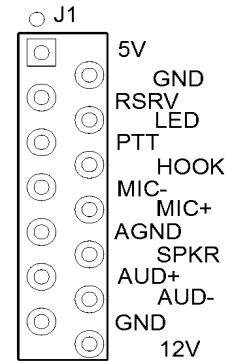
Разъем IDC14 (вид сверху)
