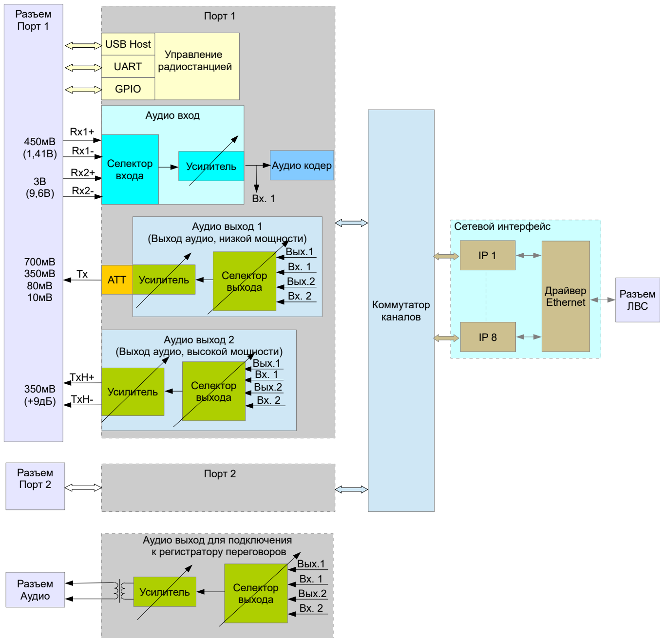
Рис. 2.2 Блок схема интерфейсов Порт 1 и 2, Аудио и ЛВС контроллера М-310.
