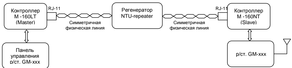
Рис. 6. Схема соединения контроллеров с использованием NTU регенератора
