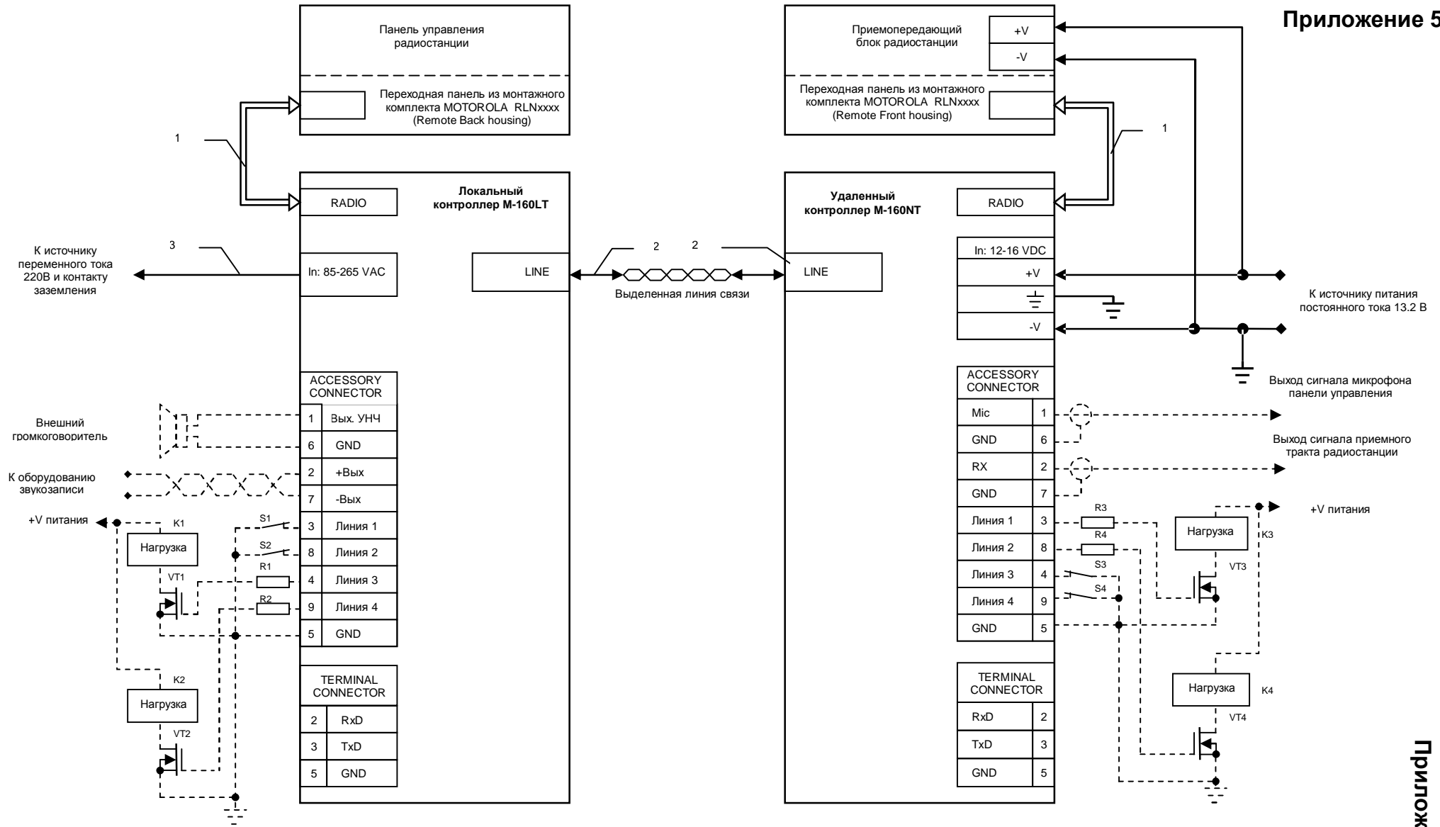
Схема подключения панели управления и приемопередающего блока радиостанции к контроллерам системы M-160
